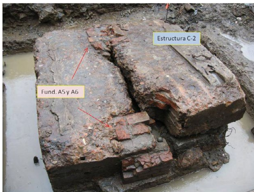
Figura 10. Estructura C, levantada sobre fundaciones A5 y A6, construidas con anterioridad.
