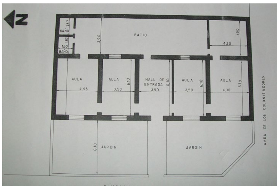
Figura 9. Plano de la planta baja de la Casa de la Colonia. En el mismo, falta el trazo de la escalera que da acceso a la planta superior, la misma se encuentra en el hall. Plano obtenido de la Secretaría de Obras Públicas y Planeamiento Municipalidad de Esperanza.
